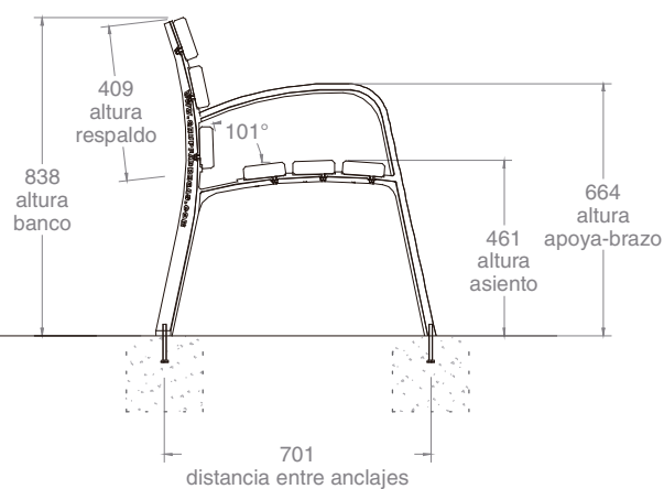
vista lateral 1:20
