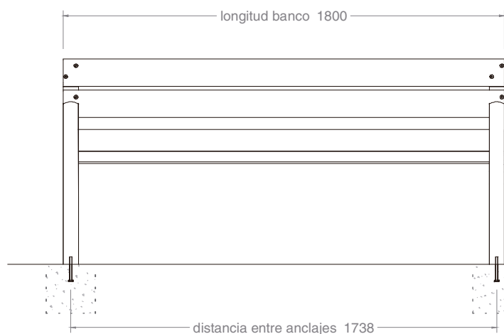
vista frontal 1:20
