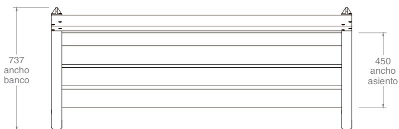
vista en planta 1:20
