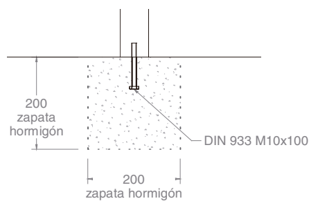
DETALLE ANCLAJE 1:10
