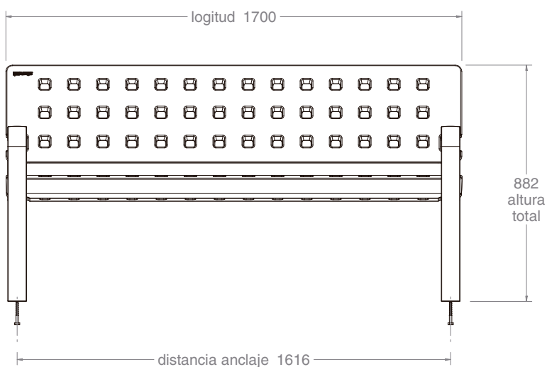
vista frontal 1:20
