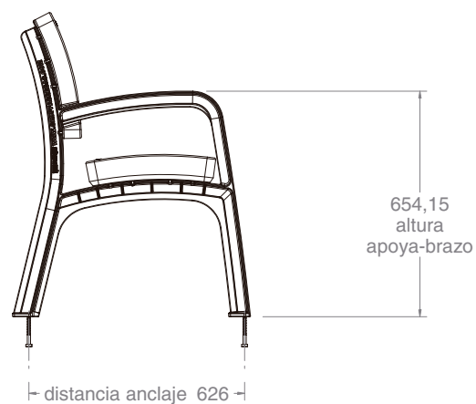
vista lateral 1:20
