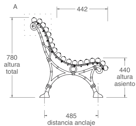
vista lateral 1:20
