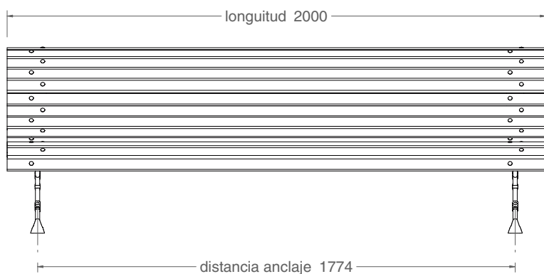
vista alzado 1:20
