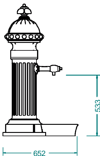
vista lateral 1:20
