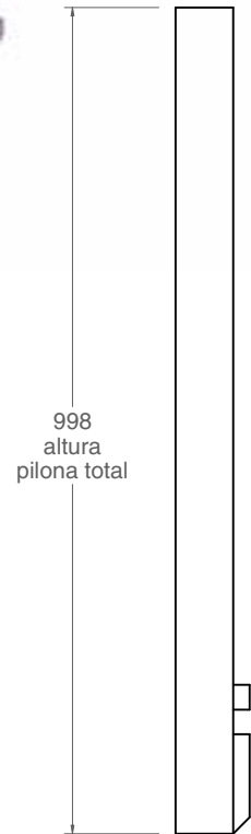
vista alzado pilona 1:10
