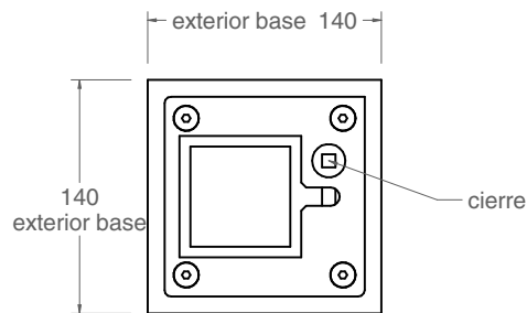
vista en planta base 1:5
